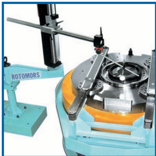
Stazione di preparazione e controllo con braccio snodato porta comparatore
